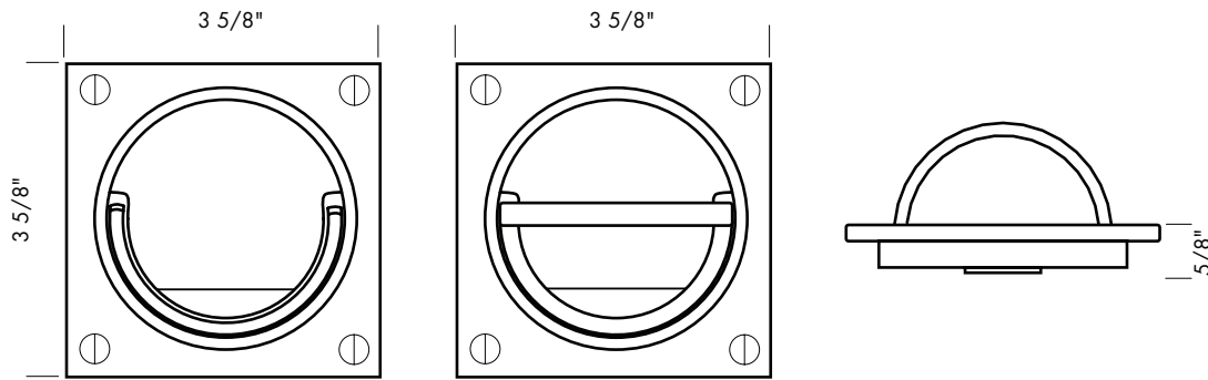
SQFP-358
